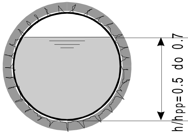
fekalni kanal
